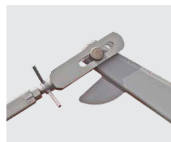
Braços reguláveis para articulação dos montantes. Adjustable bars for the articulation of the side frames. Brazos regulables para articulación de los marcos laterales (cuadros y/o cuerpos laterales).
