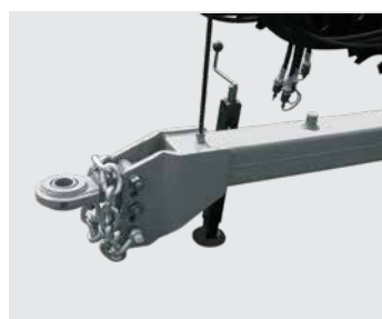
Cabeçalho regulável com correntes de segurança. Adjustable draw bar with safety chain. Lanza de enganche regulable con cadenas de seguridad.
